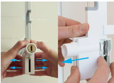
4. Schuif de behuizing eraf: zet uw duim boven de behuizing, trek de zijkanten uit elkaar, schuif de behuizing naar voren
