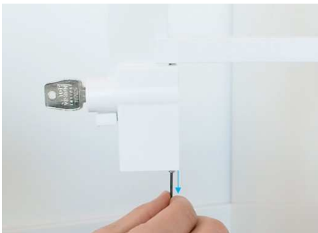
1. Draai de schroef aan de onderkant van de slot module eruit
