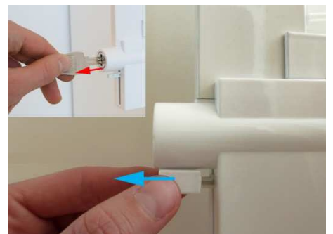
3. Haal het kapje van de locking slider eraf
