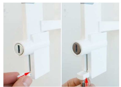
12. Plaats het kapje van de locking slider terug en schroef het weer vast
