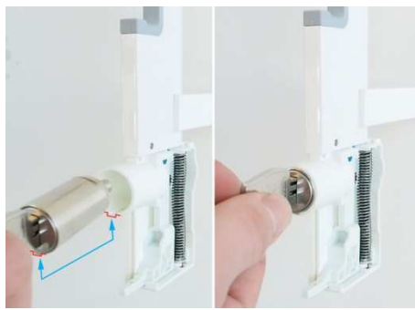
8. Schuif het nieuwe slot in de module
