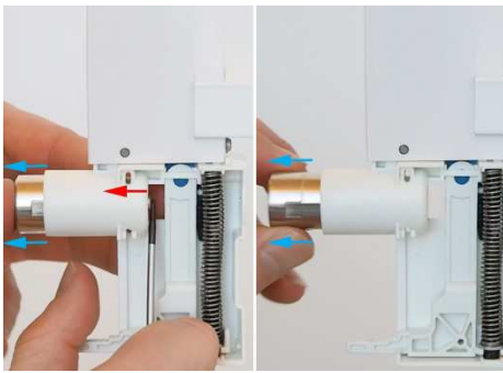
7. Duw voorzichtig het slot eruit
