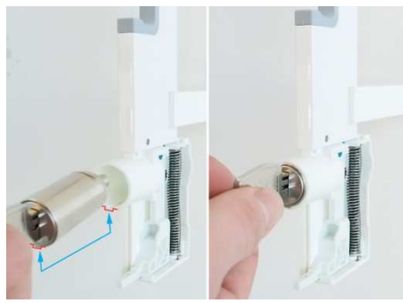
8. Coloque la nueva cerradura en su sitio como se indica
